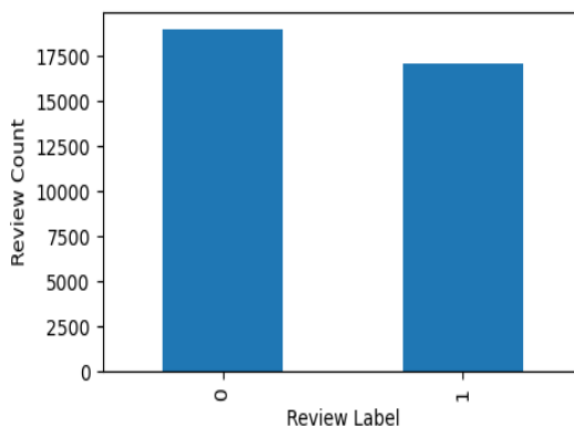
Fig. 2. Dataset Description
